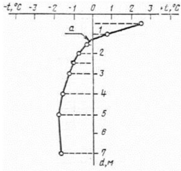
График распределения температуры t , °C, грунта по длине d , м, для одnorазовых измерений температуры
