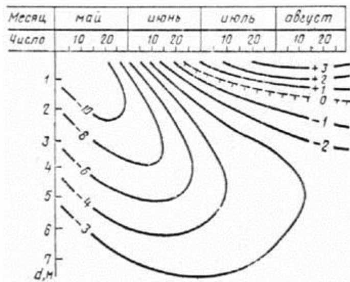
График термоизоплент по скважине № _____ за период с _____ по _____ по данным режимных (длительных) температурных наблюдений
