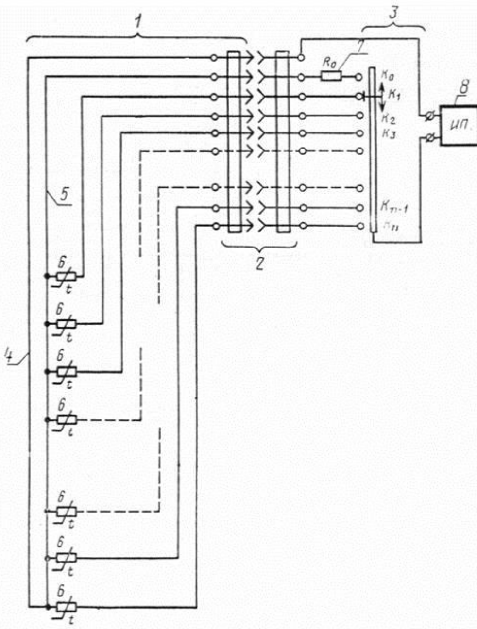
1 — гирлянда электрических термометров сопротивления; 2 — разъем; 3 — переключатель; 4 — общий провод; 5 — компенсационный провод; 6 — электрические термометры сопротивления с номиналом 100 Ом; 7 — образцовый резистор (стабилизированный манганин) с номиналом R_0 = 100 \text{ Ом} (\pm 0,01\%) ; 8 — измерительный прибор
