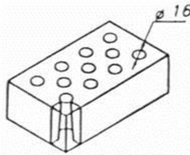
Рисунок А13 — Кирпич с 11 сквозными отверстиями (пустотность 8,2 %)
