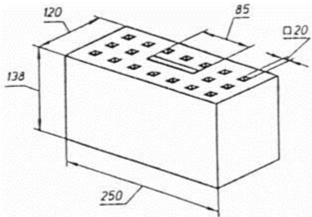
Рисунок А22 — Камень с квадратными пустотами (пустотность 33 %)
