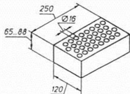
Рисунок А2 — Кирпич с 32 пустотами (пустотность 22 %)
