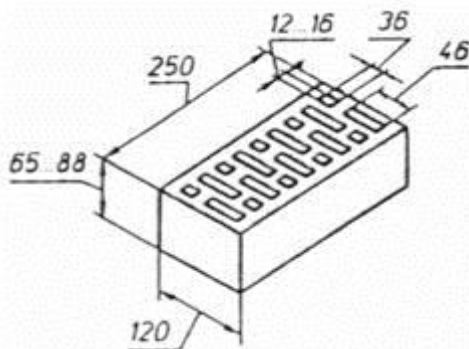
Рисунок А4 — Кирпич с 18 пустотами (пустотность 29 %, 38 %)
