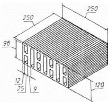
Рисунок А17 — Камень с 11 горизонтальными пустотами
