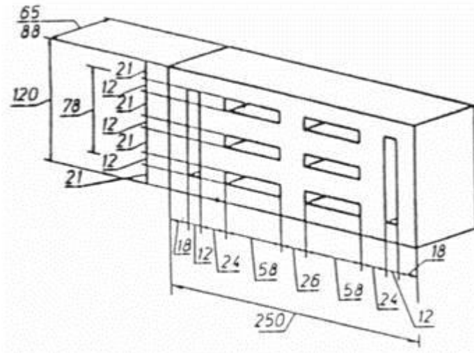
Рисунок А20 — Кирпич с 8 пустотами (пустотность 20 %)
