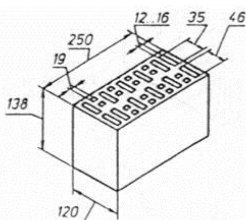
Рисунок А9 — Камень с 28 пустотами (пустотность 32 %, 42 %)
