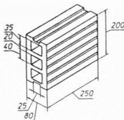
Рисунок А18 — Камень с 3 горизонтальными пустотами
