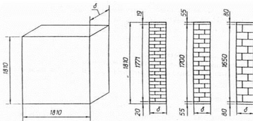
a — фрагмент кладки в аксонометрии
