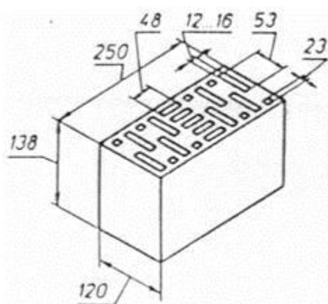
Рисунок А8 — Камень с 21 пустотами (пустотность 34 %, 45 %)
