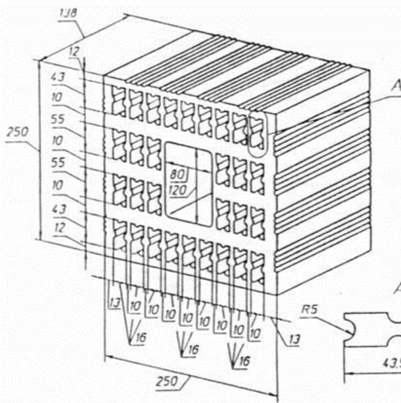
Рисунок А19 — Камень с 30 пустотами и пустотой для захвата при кладке (пустотность 45 %)
