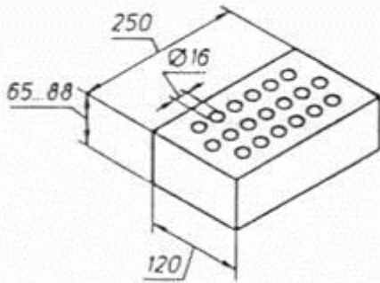
Рисунок А1 — Кирпич с 19 пустотами (пустотность 13 %)
