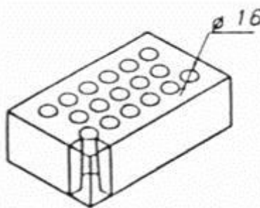
Рисунок А14 — Кирпич с 17 сквозными отверстиями (пустотность 12,7 %)
