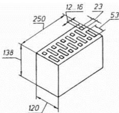
Рисунок А7 — Камень с 18 пустотами (пустотность 27 %, 36 %)
