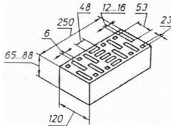
Рисунок А3 — Кирпич с 21 пустотами (пустотность 34 %, 45 %)
