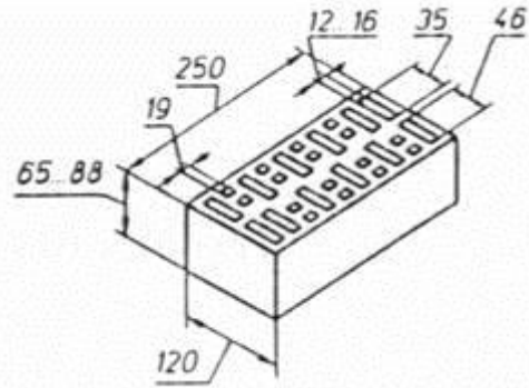
Рисунок А5 — Кирпич с 28 пустотами (пустотность 32 %, 42 %)
