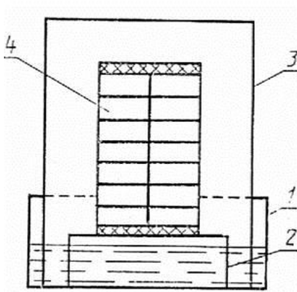
1 - сосуд-основание с водой; 2 - подставка для укладки образцов; 3 - колпак; 4 - контейнер с образцами изделий
