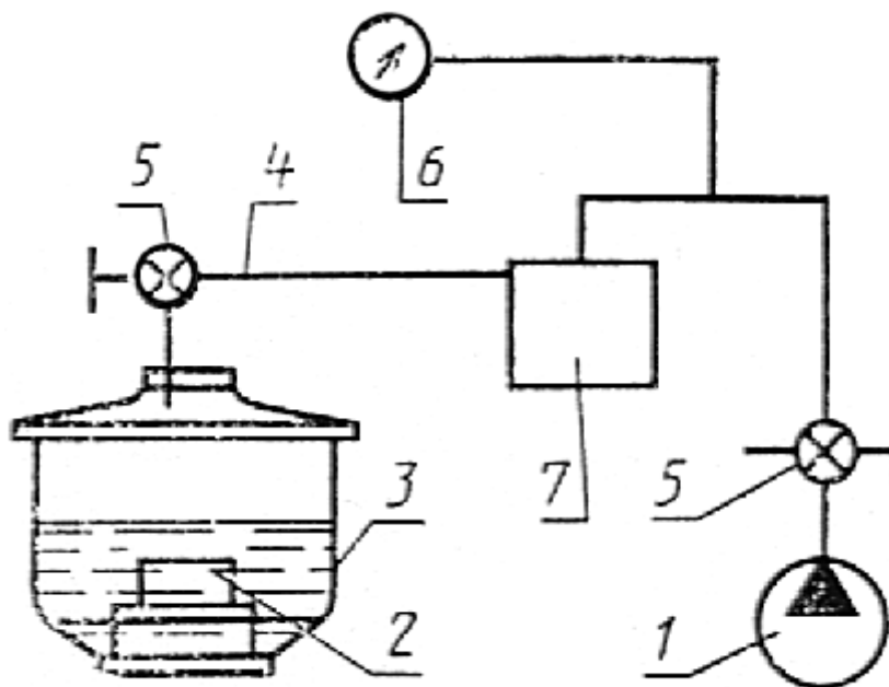
Схема установки для определения водопоглощения под вакуумом
