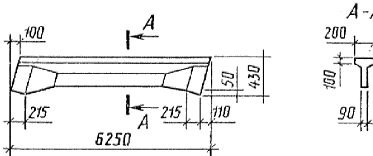
Балка типоразмера 1БСО6 (серия 1.862.1-5)
