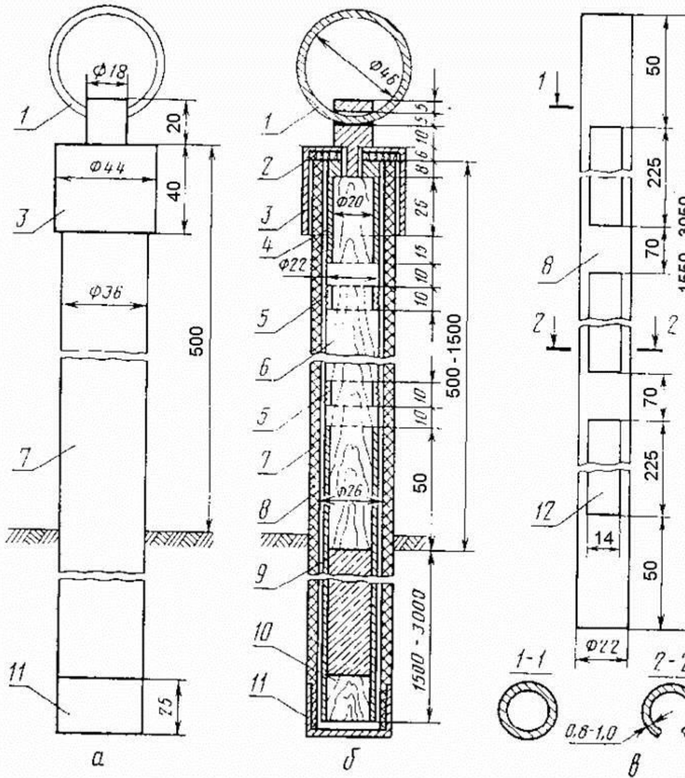
а - общий вид; б - продольный разрез; в - металлическая трубка; 1 - металлический стержень с кольцом для удержания мерзлотомера в строго фиксированном положении; 2 - войлочная прокладка; 3 - металлический колпачок для закрытия обсадной трубки; 4 - металлическая обойма стержня; 5 - войлочная обертка, стянутая проволокой; 6 - деревянный стержень; 7 - обсадная фенопластмассовая (эбонитовая) трубка; 8 - трубка из нержавеющей стали, заполняемая глинистым грунтом; 9 - влажный глинистый грунт - наполнитель металлической трубки; 10 - деревянная пробка; 11 - металлическая насадка; 12 - прорези
