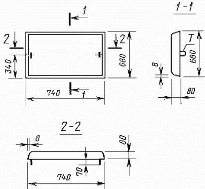
T - подъемная технологическая петля Черт. 3
