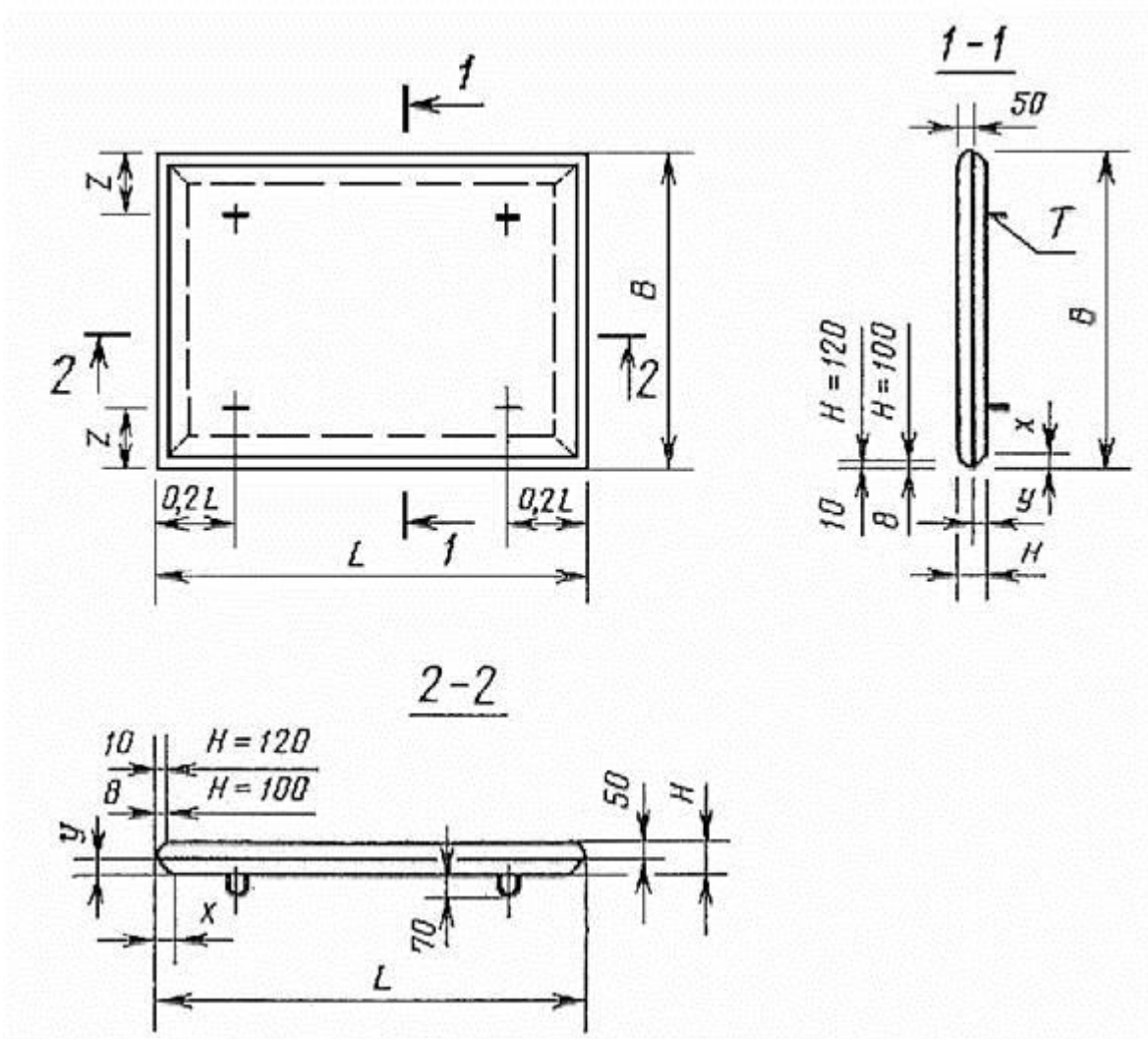
T - подъемная технологическая петля Черт. 2
