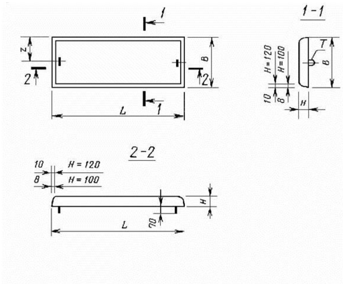
Т - подъемная технологическая петля Черт.1
