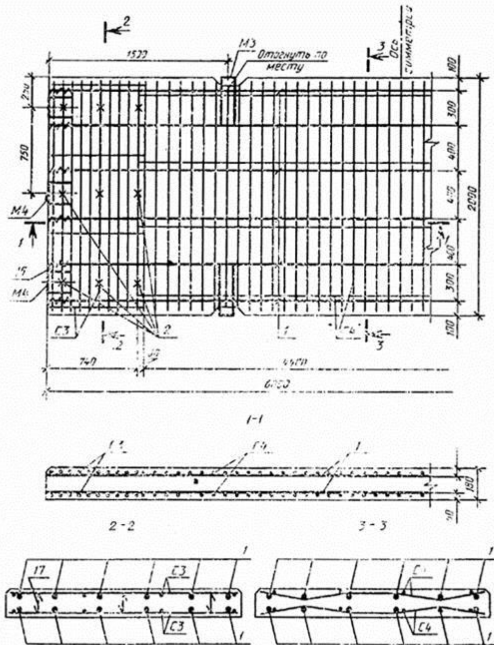
1 — напрягаемая арматура; 2 — крепление сеток С3 Черт. 1
